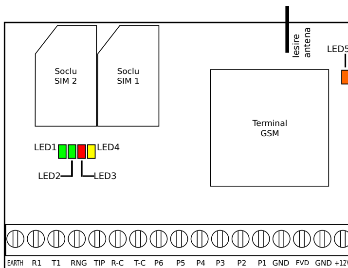
Figura 1: Diagrama de conectare a modului rev. 5
